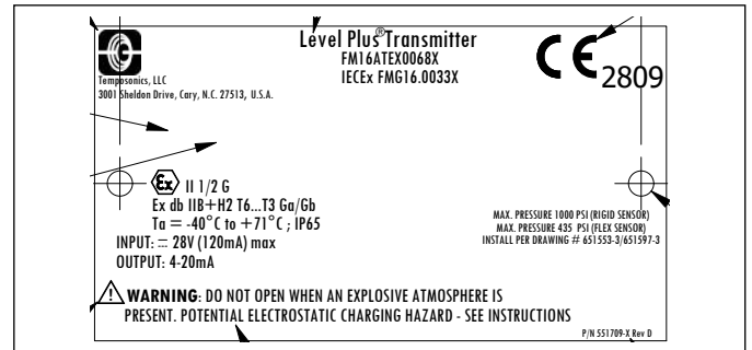
그림39: 방염, ATEX/IECEx 라벨, 아날로그, 듀얼 캐비티 하우징
