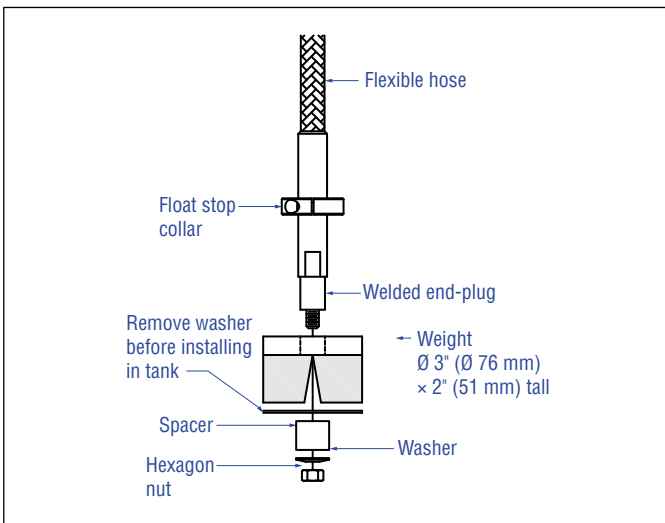
그림7: 하단 고정 자석
