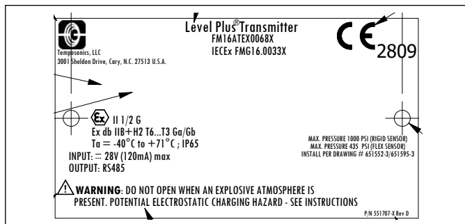
그림38: 방염, ATEX and IECEx 라벨, Modbus 듀얼 캐비티 하우징
