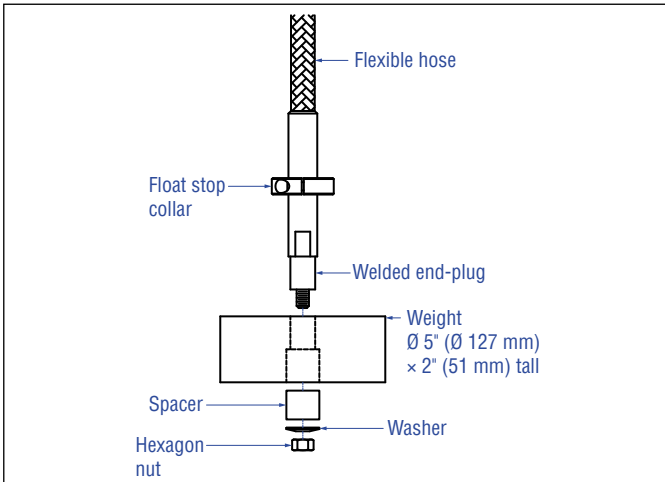
그림6: 하단 고정 추
