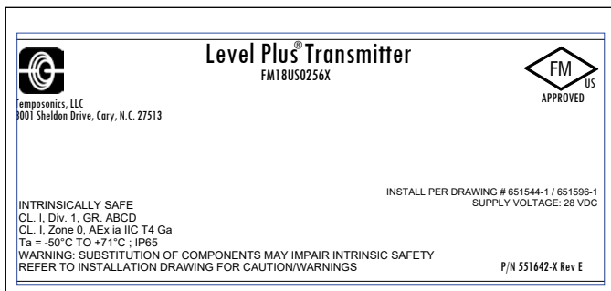
그림 15: 본질 안전 FM 라벨, 아날로그, 듀얼 챔버 하우징
