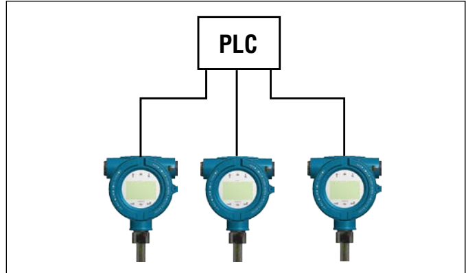
그림9: 포인트 투 포인트 토폴로지
