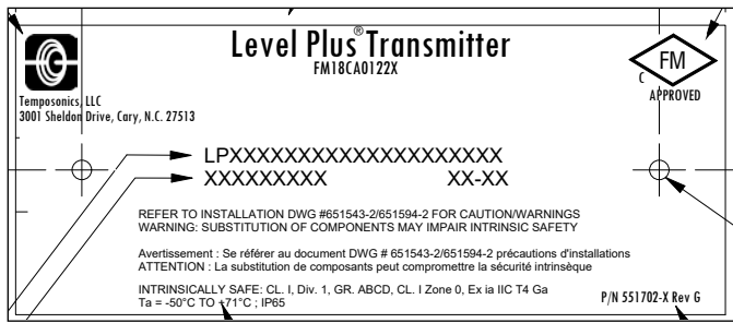
그림22: 본질 안전 FMC 라벨, Modbus 듀얼 캐비티 하우징
