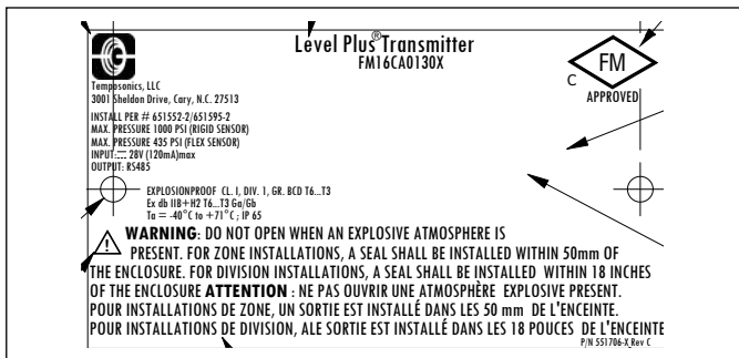
그림28: 방폭, FMC 라벨, Modbus 듀얼 캐비티 하우징
