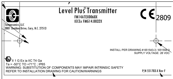
그림34: 본질 안전 ATEX/IECEx 라벨, Modbus, 듀얼 챔버티 하우징
