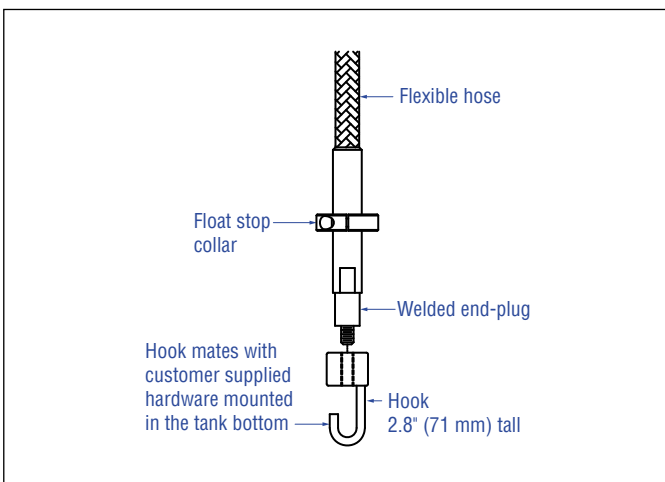
그림8: 하단 고정 후크
