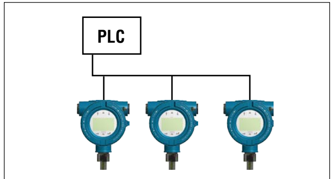
그림10: 스퍼 토폴로지 사용 버스
