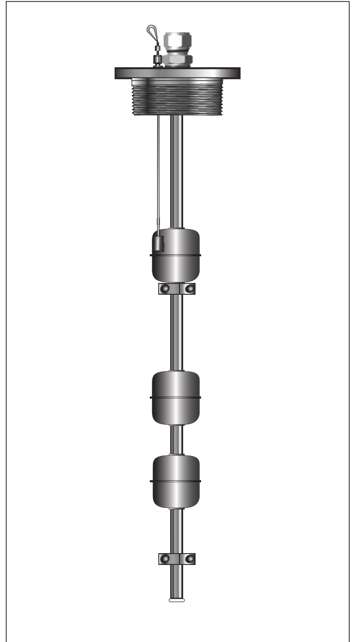
그림3: 외부 파이프 구성
