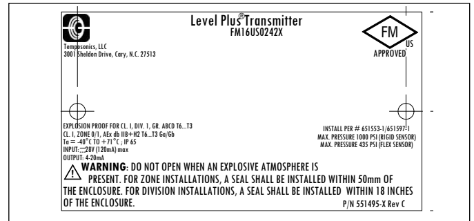
그림19: 방폭, FM 라벨, 아날로그, 듀얼 캐비티 하우징
