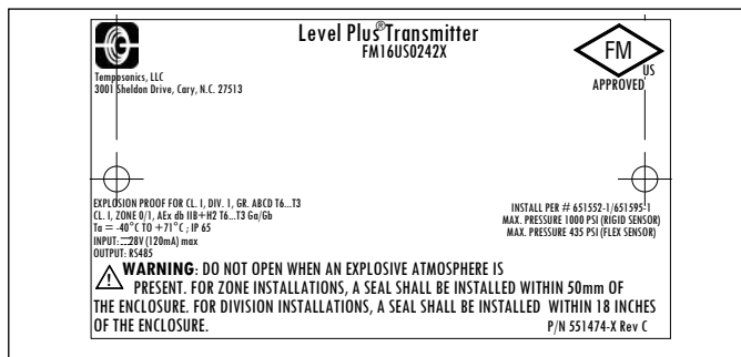
그림18: 방폭, FM 라벨, Modbus 듀얼 캐비티 하우징
