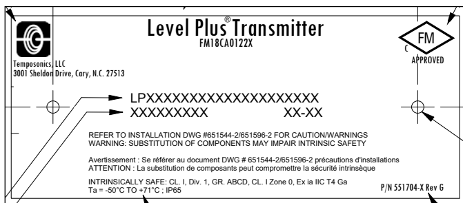
그림23: 본질 안전 FMC 라벨, 아날로그, 듀얼 캐비티 하우징
