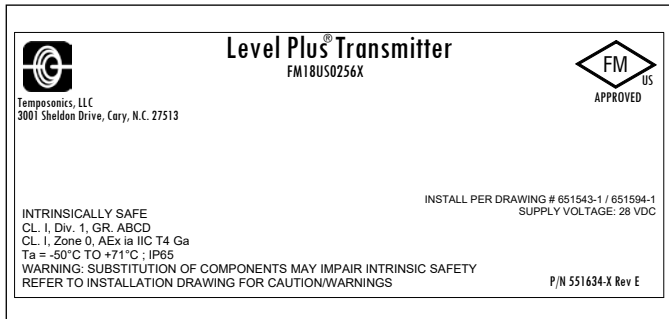
그림 14: 본질 안전 FM 라벨, Modbus, 듀얼 챔버 하우징
