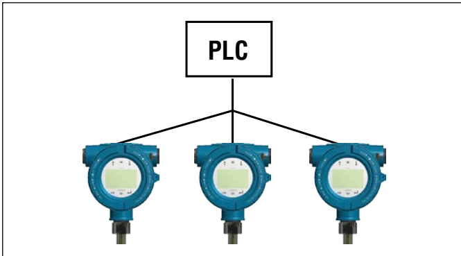
그림11: 트리 토폴로지
