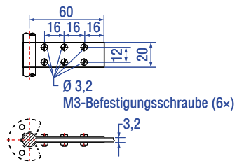
Befestigungslasche ArtikeInr. 561 481
