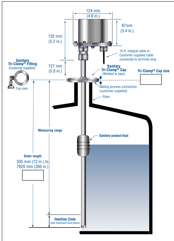
图10: 管子三夹头安装
