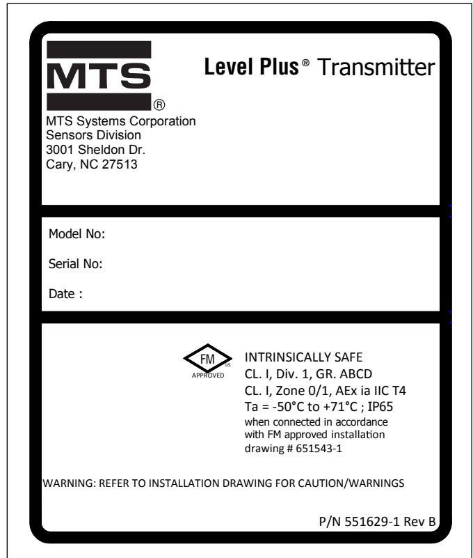
图16: 本质安全型FM标签, HART®, NEMA外壳
