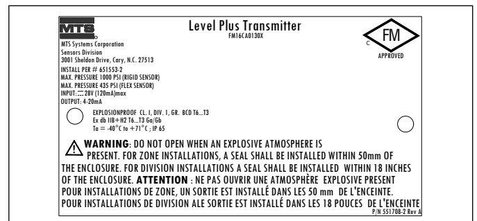
图44: 防爆型, FMC标签, HART®, 外壳选型D、E
