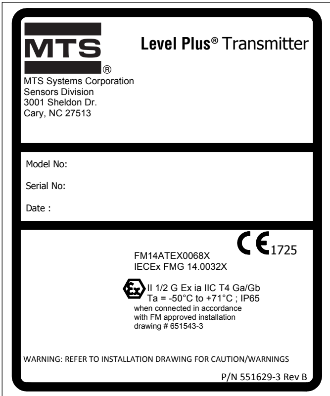
图51: 本质安全型FMC标签, Modbus和DDA, NEMA外壳
