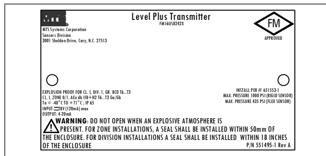
图26: 防爆型, FM标签, HART®, 外壳选型D、E
