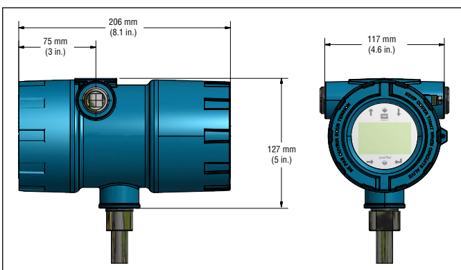
图3: 双腔外壳
