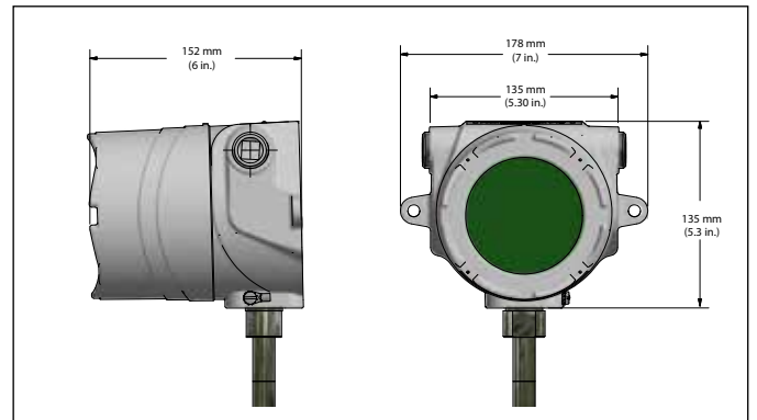
図 4 : ステンレス鋼シングルキャビティハウジング
