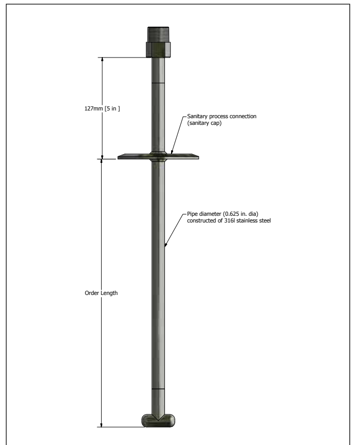
図 5 : 外パイプの構成
