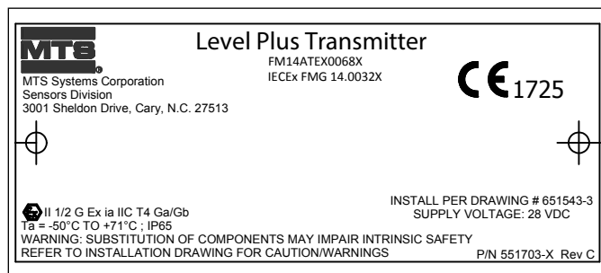
図 53 : 本質的安全 ATEX/IECEX ラベル、Modbus および DDA、シングルおよびデュアルキャパシティハウジング
