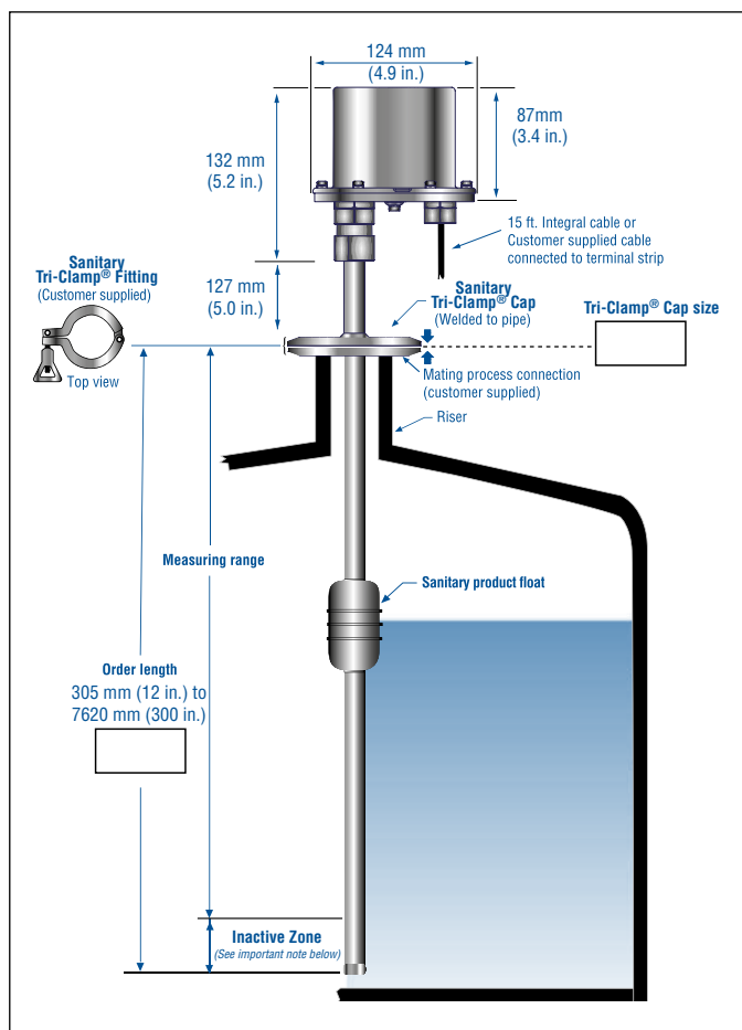
図 10 : Tri-clamp によるパイプの取り付け
