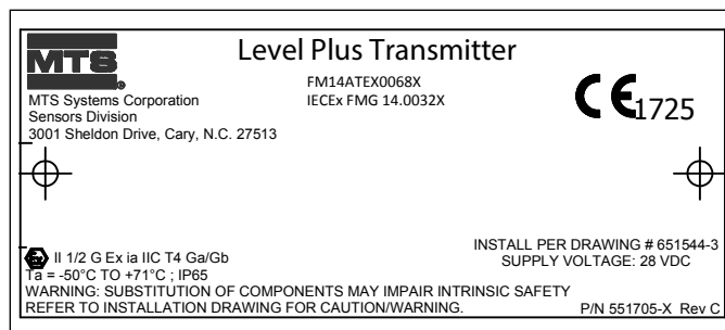
図 54 : 本質的安全 ATEX/IECEX ラベル、Modbus および DDA、シングルおよびデュアルキャパシティハウジング
