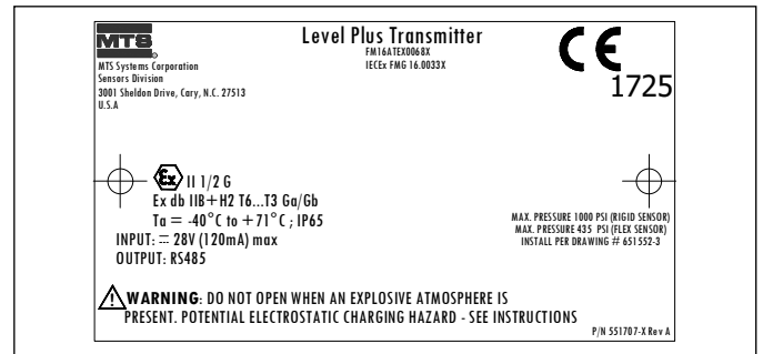
図 59 : 防災、ATEX および IECEx ラベル、Modbus または DDA ハウジングオプション D、E、G、H、L
