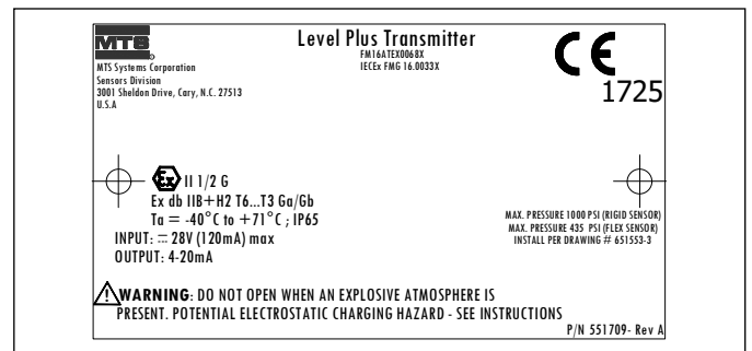
図 60 : 防災、ATEX および IECEx ラベル、HART® ハウジングオプション D、E、G、H、L
