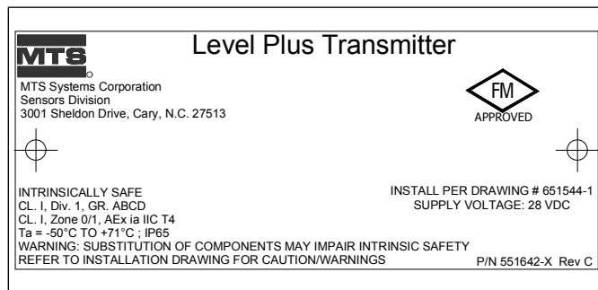
図 18 : 本質的安全 FM ラベル、HART、シングルまたはデュアルキャパシティハウジング
