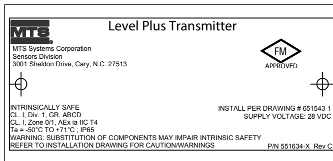
図 17 : 本質的安全 FM ラベル、Modbus または DDA、シングルまたはデュアルキャパシティハウジング
