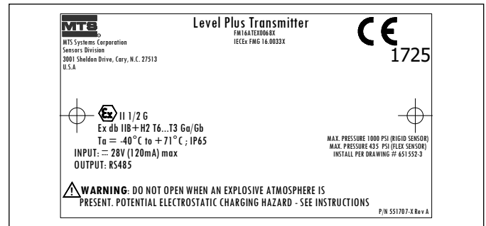
Fig. 59: Etiqueta ATEX e IECEx, à prova de chamas, Modbus ou DDA, invólucro D, E, G, H ou L
