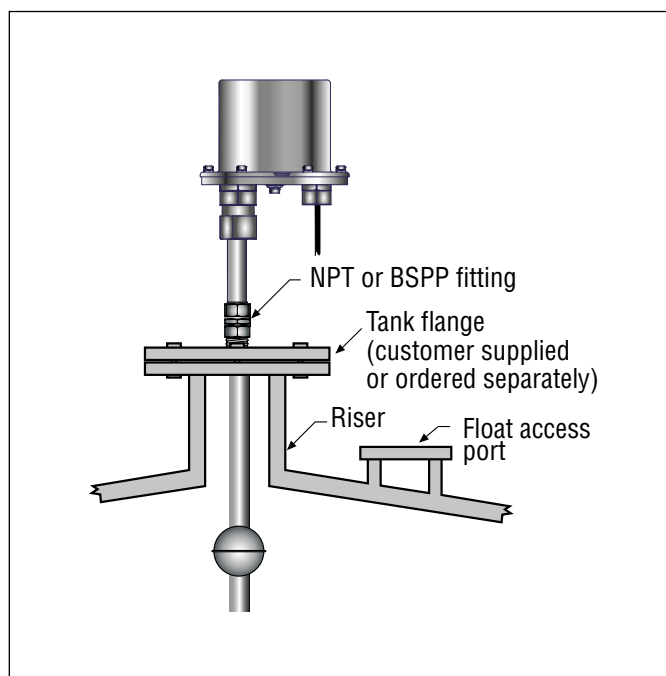
Fig. 8: Montagem em flange roscado para haste flexível
