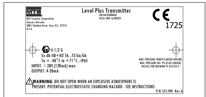
Fig. 60: Etiqueta ATEX e IECEx, à prova de chamas, HART®, invólucro D, E, G, H ou L
