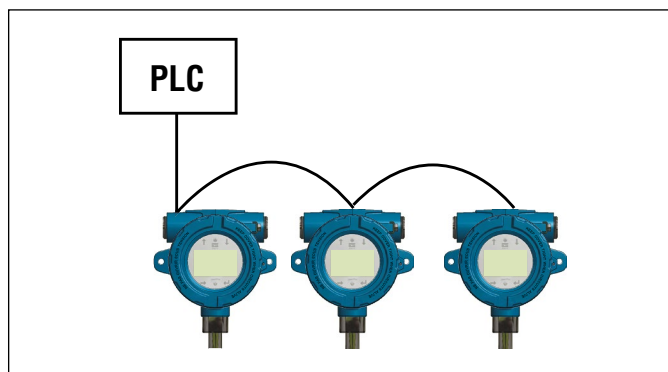
Fig. 13: Topologia Daisy-chain (encadeamento)
