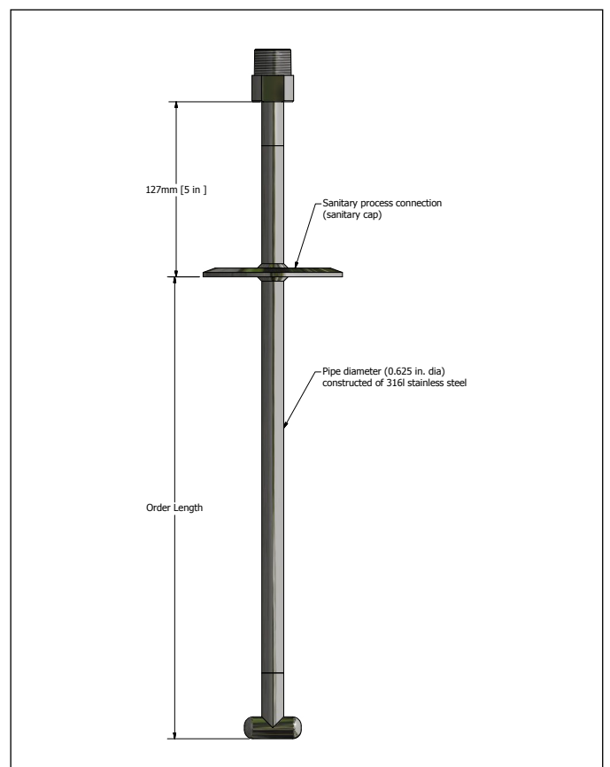
Fig. 5: Configuração da haste externa
