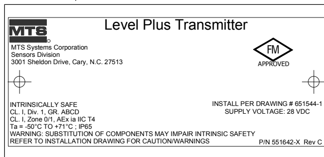
Fig. 18: Etiqueta FM intrinsecamente segura, HART®, invólucro com cavidade única ou dupla
