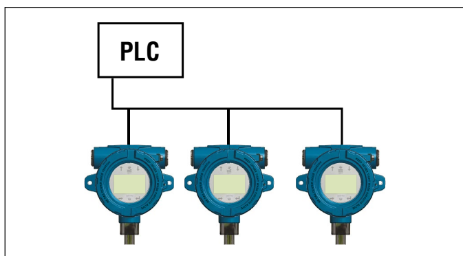
Fig. 11: Topologia barramento com antena
