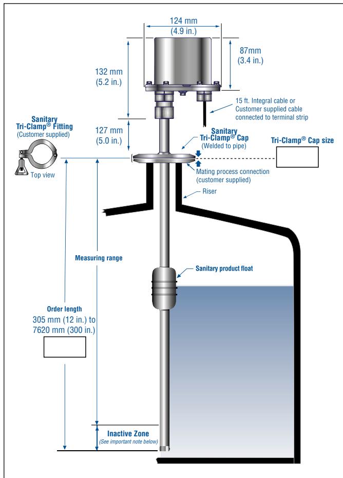
Fig. 10: Montagem da haste com braçadeira Tri-clamp
