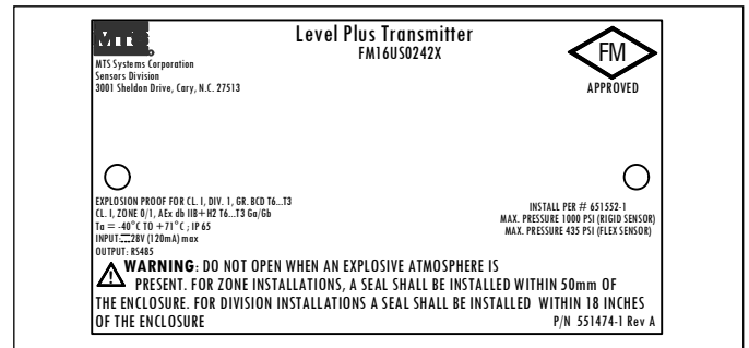
Fig. 23: Etiqueta FM, à prova de explosão, Modbus ou DDA, opções de invólucro G, H ou L
