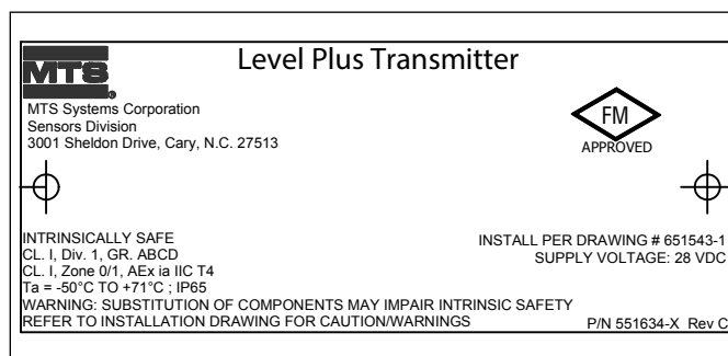
Fig. 17: Etiqueta FM intrinsecamente segura, Modbus ou DDA, invólucro com cavidade única ou dupla
