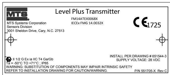
Fig. 54: Etiqueta ATEX/IECEx intrinsecamente segura, Modbus e DDA, invólucro com cavidade única ou dupla
