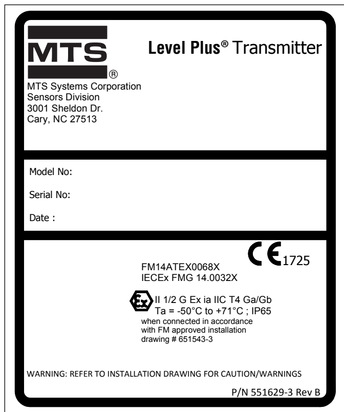
Fig. 51: Etiqueta FMC intrinsecamente segura, Modbus e DDA, invólucro NEMA
