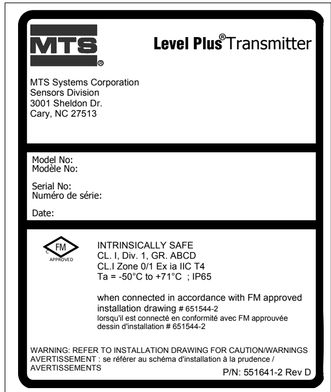
Fig. 32: Etiqueta FMC intrinsecamente segura, HART®, invólucro NEMA
