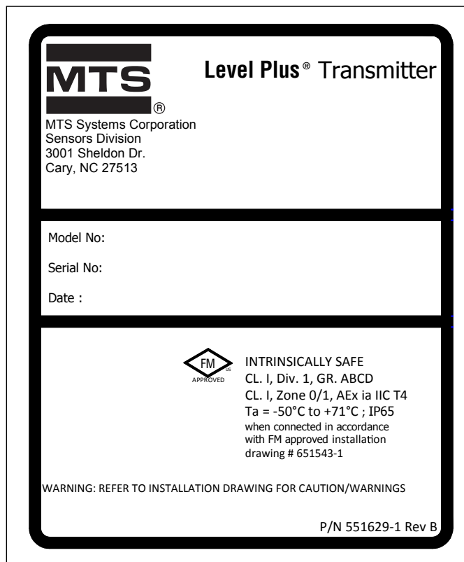
Fig. 16: Etiqueta FM intrinsecamente segura, invólucro HART®, NEMA
