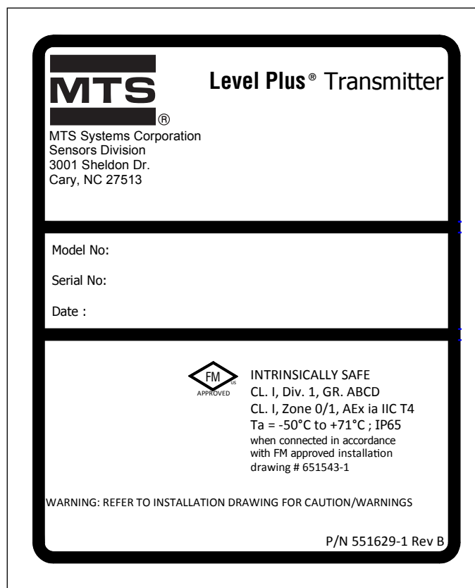
Fig. 15: Etiqueta FM intrinsecamente segura, Modbus ou DDA, invólucro NEMA
