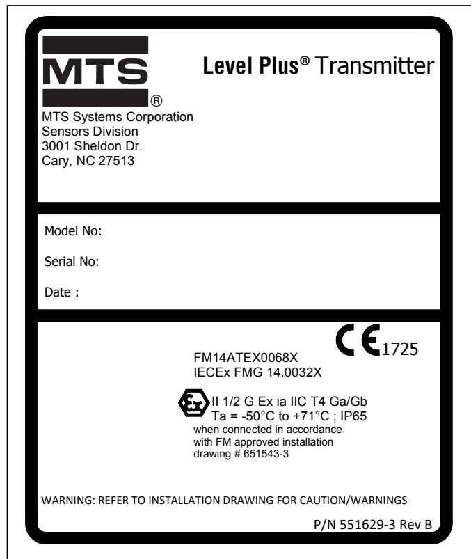
Fig. 52: Etiqueta ATEX/IECEx intrinsecamente segura, Modbus e DDA, invólucro NEMA
