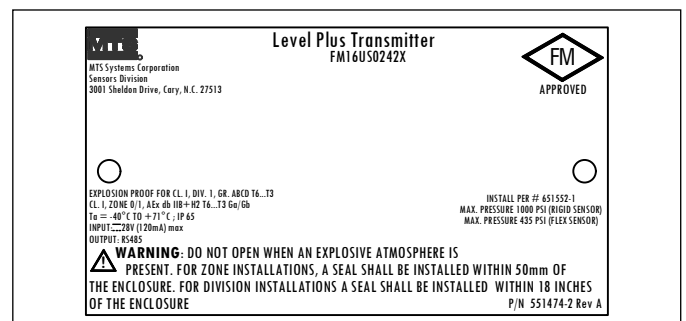
Fig. 24: Etiqueta FM, à prova de explosão, Modbus ou DDA, opções de invólucro D, E
