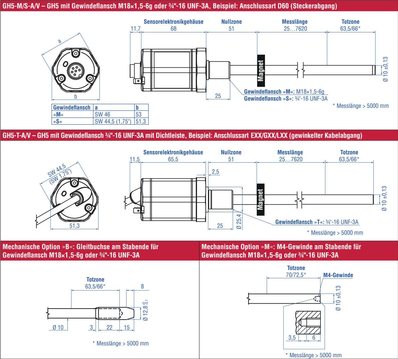
Abb. 2: Temposonics® GH5 mit Ringmagnet
