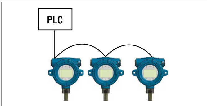
그림13: 데이지 체인 토폴로지
