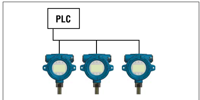
그림11: 스퍼 토폴로지 사용 버스
