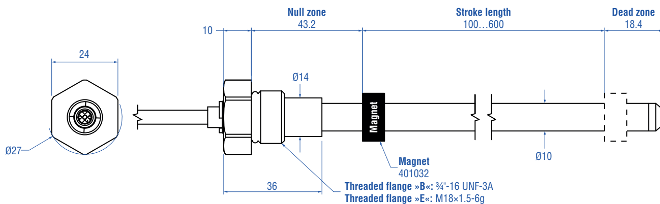
Fig. 3: Temposonics® MH-Series SLIM Sensor
