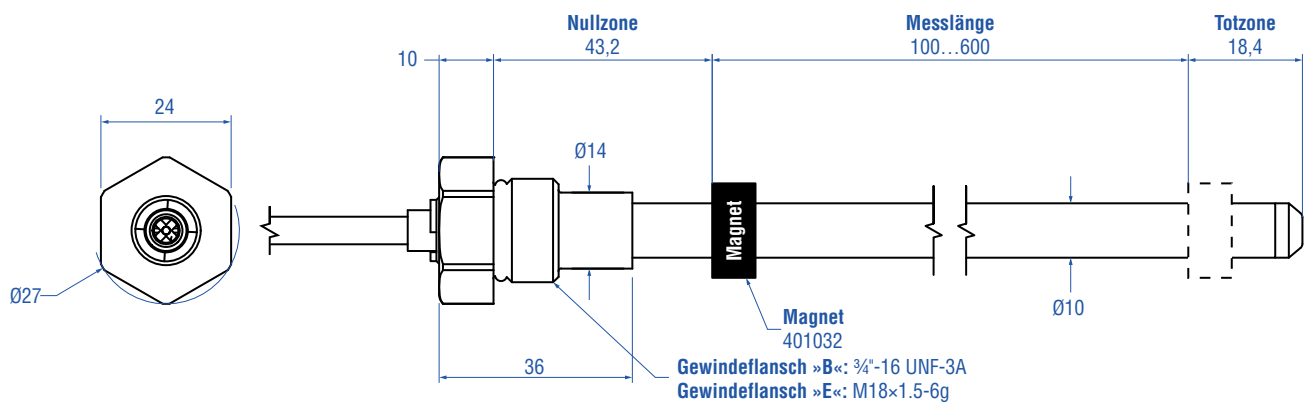
Fig. 3: Temposonics® MH-Serie SLIM Sensor
