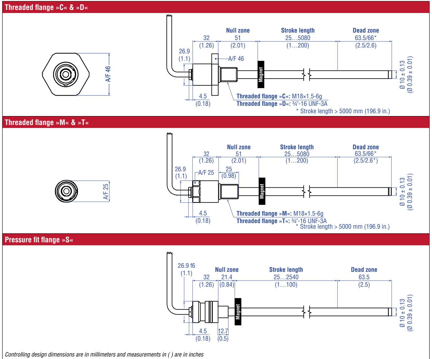
Fig. 2: Temposonics® RD5 sensor rod flange types
