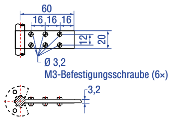
Befestigungslasche ArtikeInr. 561 481
