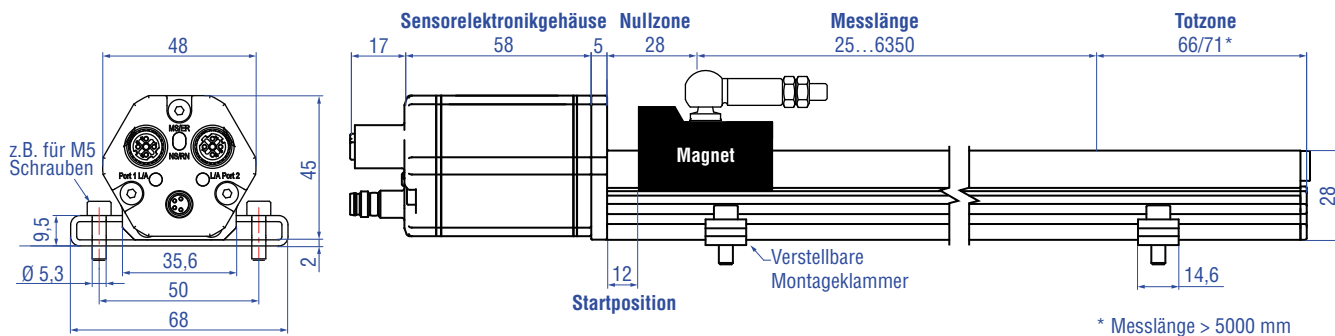
Abb. 3: Temposonics® RP5 mit U-Magnet und Magnetschlitten
