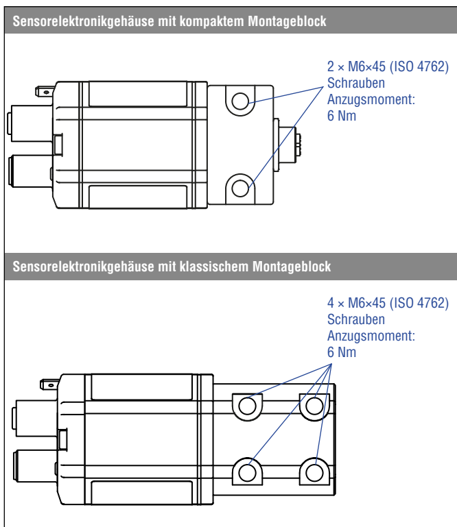
Abb. 47: Montage des RD5-Sensorelektronikgehäuses
