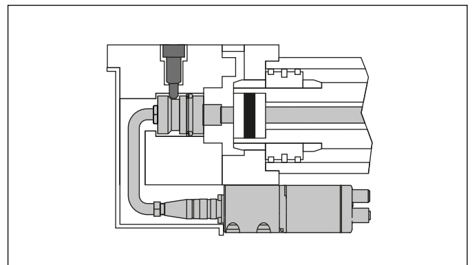
Abb. 49: RD5 mit Seitenanschluss
