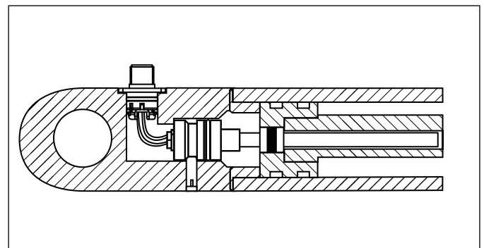
Abb. 52: M12-Vierkant-Flanschstecker im Zylinder verbaut
