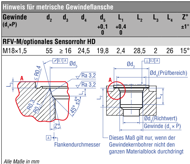
Abb. 34: Hinweis für metrischen Gewindeflansch M18×1,5-6g in Anlehnung an DIN ISO 6149-1
