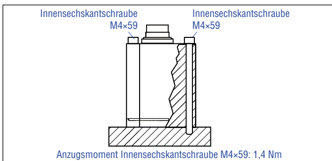
Abb. 30: Befestigung mittels Innensechskantschrauben M4×59
