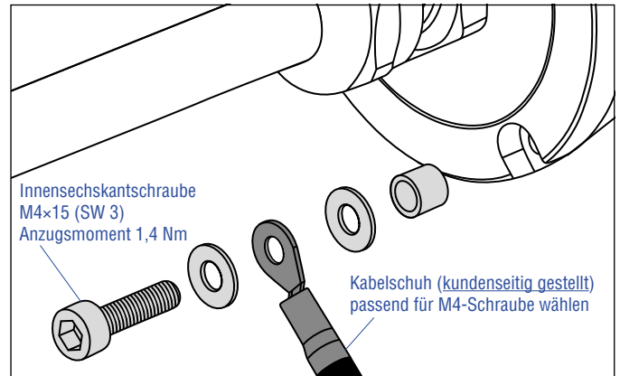
Abb. 96: Installationsbeispiel zur Erdung eines RM5-Sensors
