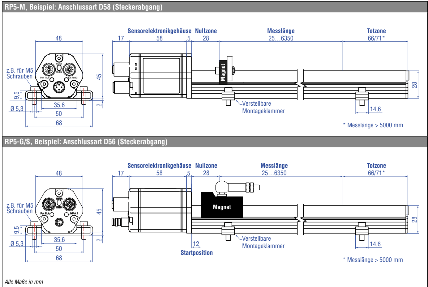
Abb. 3: Temposonics® RP5 mit U-Magnet/Magnetschlitten
