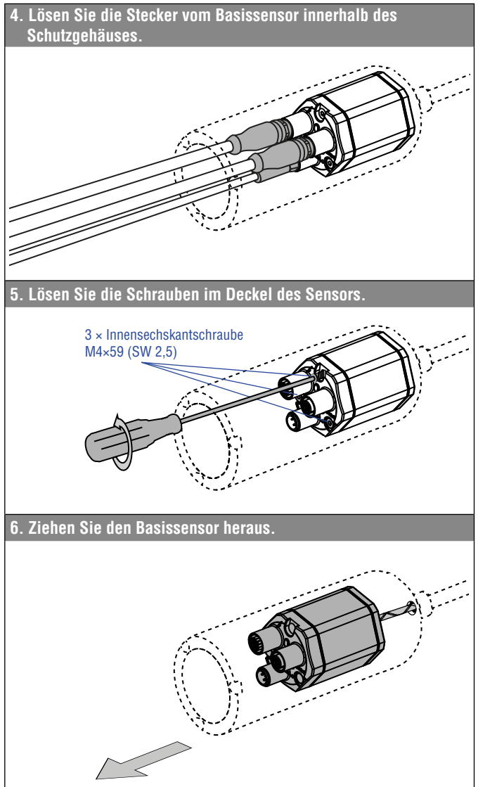
Abb. 92: Austausch des Basissensors beim Modell RM5, Teil 2
