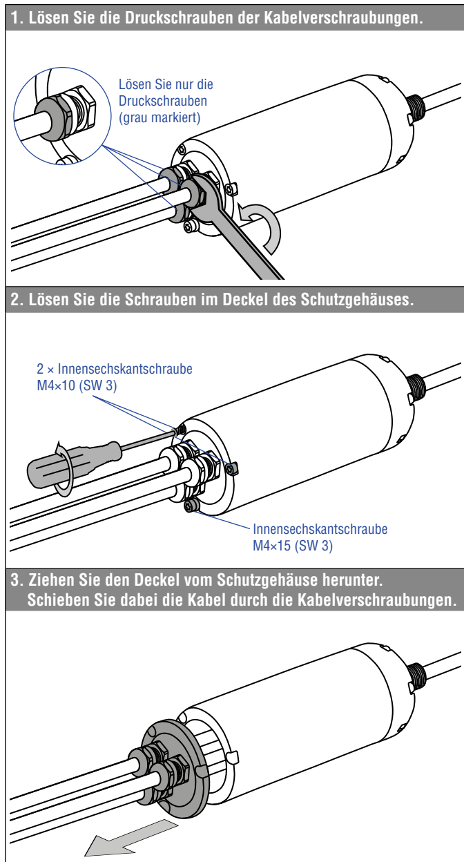
Abb. 91: Austausch des Basissensors beim Modell RM5, Teil 1
