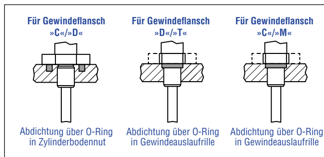
Abb. 43: Möglichkeiten der Abdichtung
