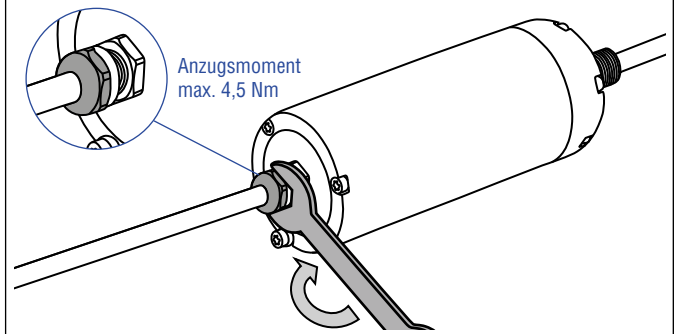
Abb. 97: Austausch des Basissensors beim Modell RM5, Teil 4
