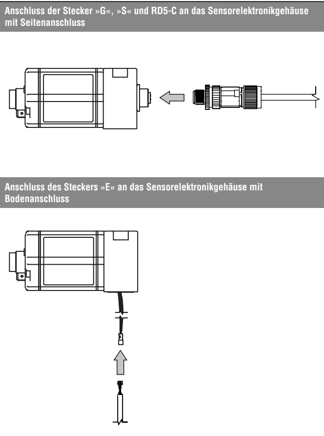
Abb. 53: Anschluss des Steckers am Kabel des RD5-Sensorstabs an die Sensorelektronik
