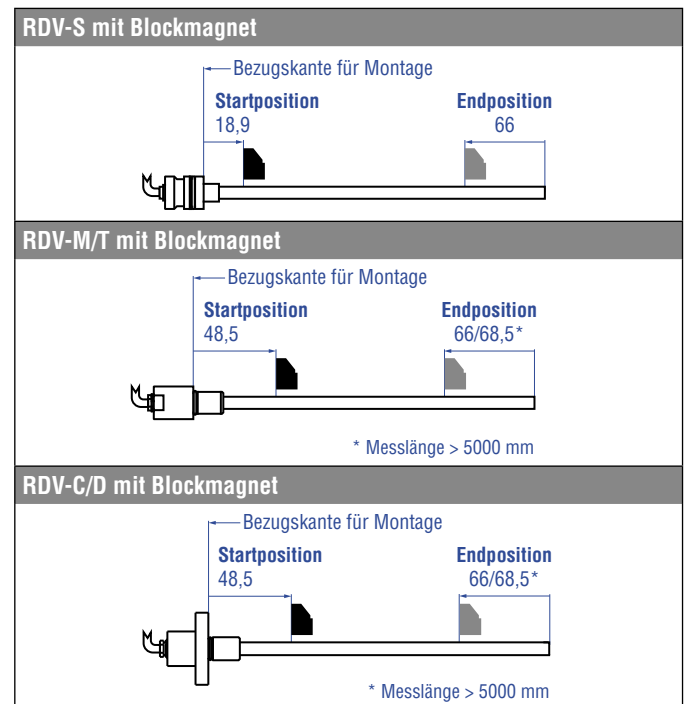
Abb. 81: Start- und Endpositionen der Magnete für RDV mit Blockmagnet
