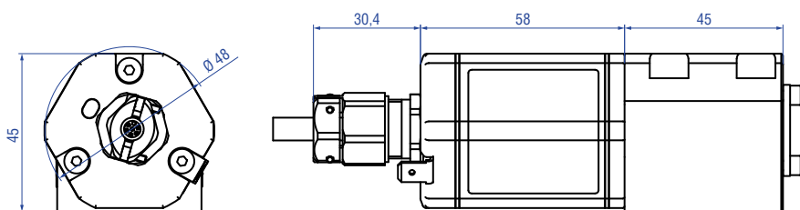
Abb. 57: Temposonics® RDV-Sensorelektronikgehäuse, Teil 2
