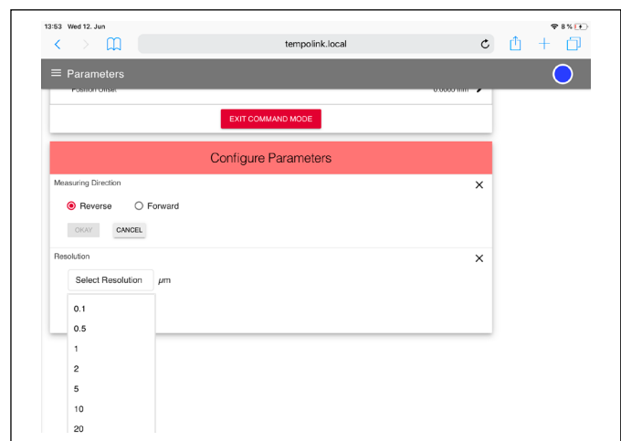
Abb. 126: Konfiguration der SSI-Parameter
