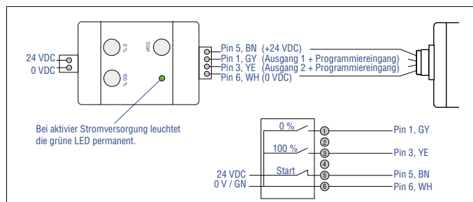
Abb. 126: Hand-Programmiergerät anschließen
